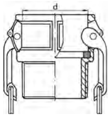
Мамка з'єднувача CAMLOCK з зовнішньою різьбою BSPT або NPT
