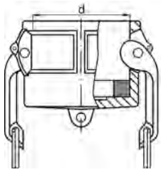
Мамка-заглушка втикової частини CAMLOCK
