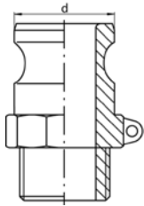
Втикова частина CAMLOCK з зовнішньою різьбою. BSPT або ж NPT
