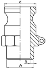
Втикова частина CAMLOCK З кінцевиком під приварку (торцеву)
