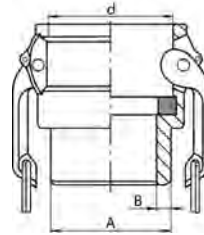
Мамка з'єднання CAMLOCK З кінцевиком під приварку (торцеву)
